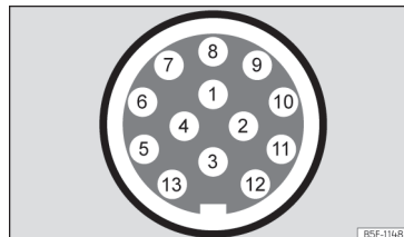
Afb. 181 Schematische weergave: toewijzing van de pinnen van het stopcontact voor de aanhangwagens.
