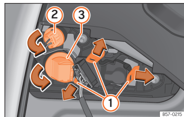
Afb. 206 Fitting uitbouwen.
