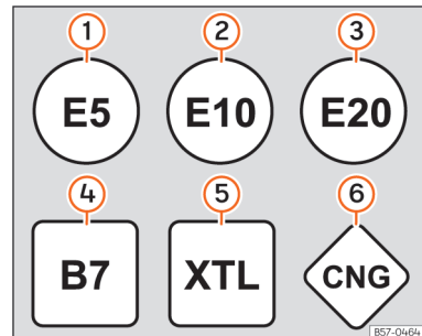
Afb. 187 Identificatie van de brandstoffen volgens richtlijn van de Europese Unie (EU) 2014/94/
