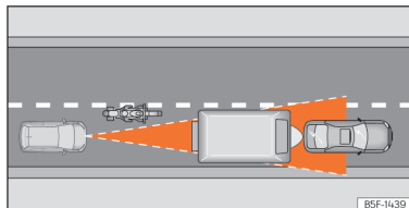
Afb. 118 Motorrijder die voor u rijdt, buiten de actieradius van de radarsensor.
