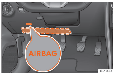
Afb. 31 Aan de bestuurderszijde: plaats van de airbag voor de knieën.
