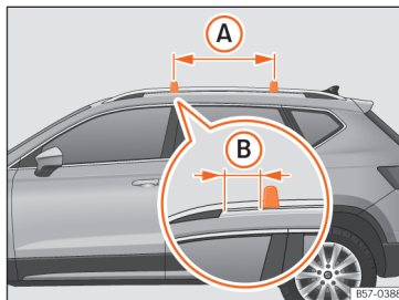
Afb. 180 Bevestigingspunten van de dwarsdragers voor het dakdragersysteem
