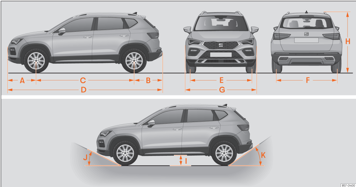
Afb. 236 Afmetingen
