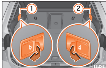
Afb. 78 In de bagageruimte: hendels voor ontgrendeling van de achterste rugleuning.
