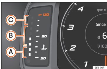
Afb. 6 Digitaal instrumentenpaneel SEAT Digital Cockpit: koelvloeistoftemperatuurmeter.
