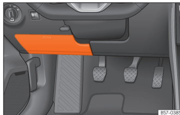
Afb. 201 In het dashboard aan bestuurderszijde: deksel van de zekeringenhouder.
