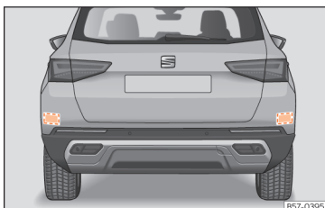
Afb. 108 Achteraanzicht van de wagen: zones van de radarsensoren.
