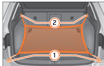
Afb. 176 In de bagageruimte: ringen ① en haken ② voor het vasthaken van de nettas.
