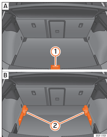
Afb. 188 Verstelbare bodem van de bagageruimte: A hoge stand; B lage stand.
