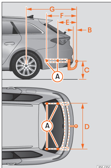
Afb. 207 Maten en bevestigingspunten voor het achteraf inbouwen van een trekhaak.
