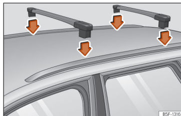
Afb. 201 Bevestigingspunten voor de reling van het dakdragersysteem (Leon Sportstourer).
