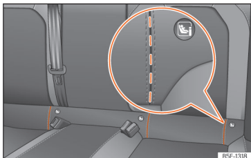
Afb. 43 Achterstoel: gestante gleuven voor toegang tot de ISOFIX/i-Size-bevestigingsbeugels.
