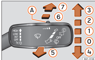
Afb. 108 Bediening van de ruitenwisser voor en achter.
