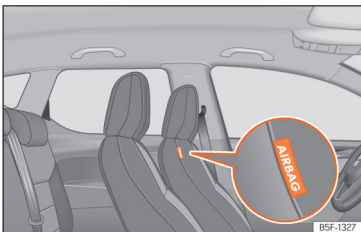
Afb. 33 In de vulling van de rugleuning van de bestuurdersstoel: centrale airbag.
