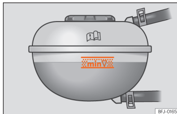
Afb. 227 In de voorruimte: markering aan het koelvloeistofexpansiereservoir.
