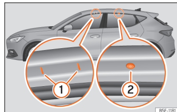
Afb. 202 Bevestigingspunten voor de reling van het dakdragersysteem (Leon).
