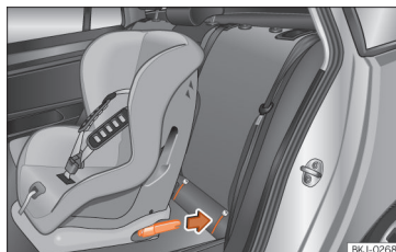
Afb. 45 Achterstoelen: plaatsing van het kinderzitje met ISOFIX-systeem.
