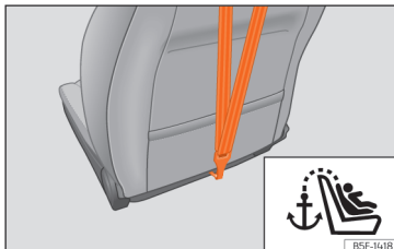
Afb. 47 Achterzijde van de rugleuning van de bijrijdersstoel: verankering voor de Top Tether-riem.
