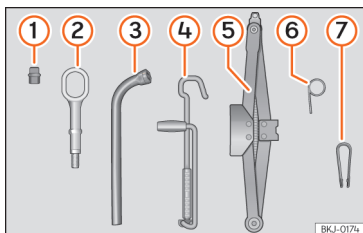
Afb. 212 Onder de afdekking van de laadvloer van de bagageruimte: wagengereedschap.
