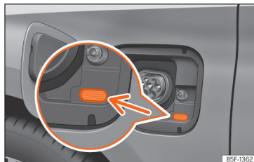
Afb. 62 Achter de acculaadklep: indicator van het laadproces.
