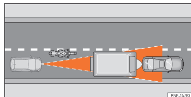
Afb. 139 Motorrijder die voor u rijdt, buiten de actieradius van de radarsensor.
