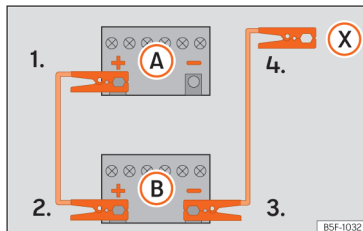
Afb. 192 Verbindingschema voor wagens zonder Start-stopsysteem.
