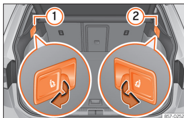
Afb. 81 In de bagageruimte: hendels voor ontgrendeling van de achterste rugleuning.
