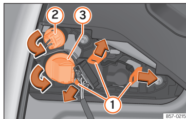
Afb. 203 Fitting uitbouwen.
