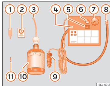
Afb. 228 Standaardweergave: inhoud van de bandenafdichtset.
