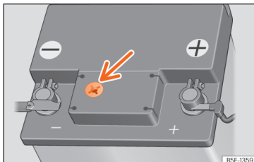
Afb. 214 Kijkglas aan de bovenzijde van de 12 volt-accu (schematische voorstelling).
