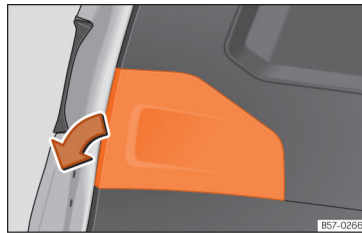
Afb. 202 Achterklep open: de afdekking verwijderen.
