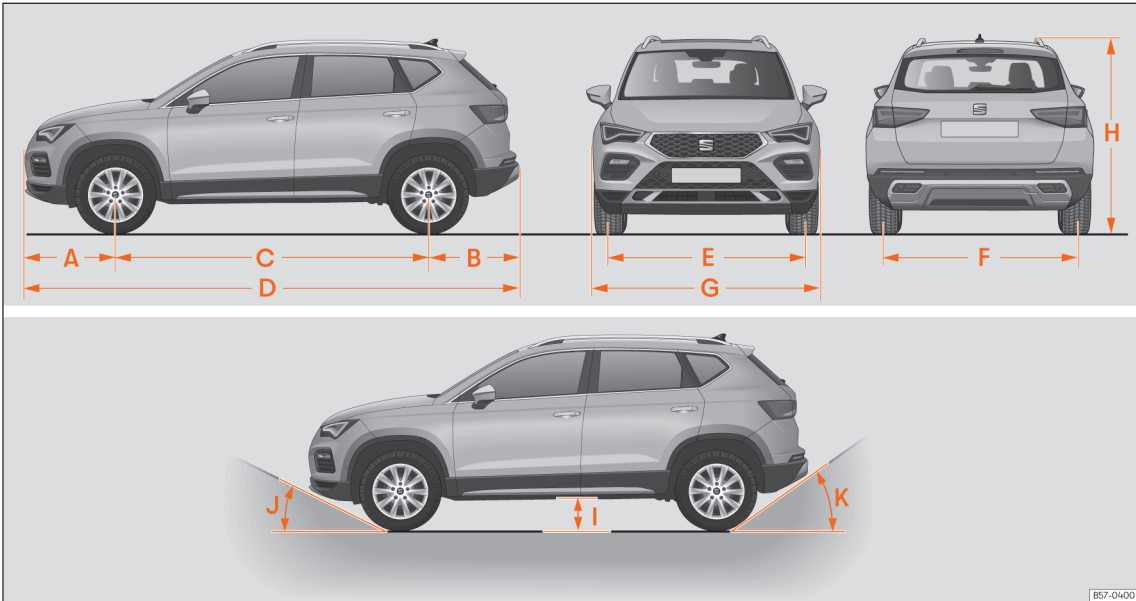
Afb. 232 Afmetingen
