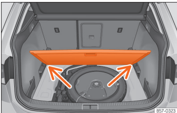
Afb. 171 Verstelbare bodem van de bagageruimte: schuine stand.
