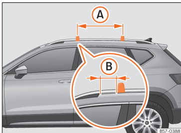
Afb. 179 Bevestigingspunten voor de reling van het dakdragersysteem
