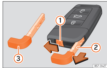
Afb. 48 Autosleutel: de nood sleutel verwijderen.
