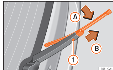
Afb. 191 Ruitenwisserblad van achterruit vervangen.
